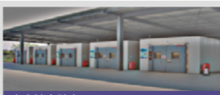
高腐蚀实验室 盐雾浓度高达 3%NaCl
